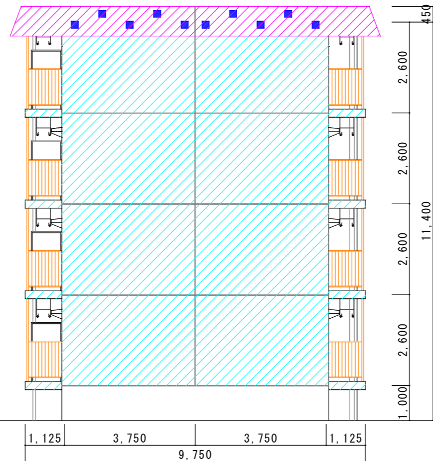
A棟・B棟 側面図
