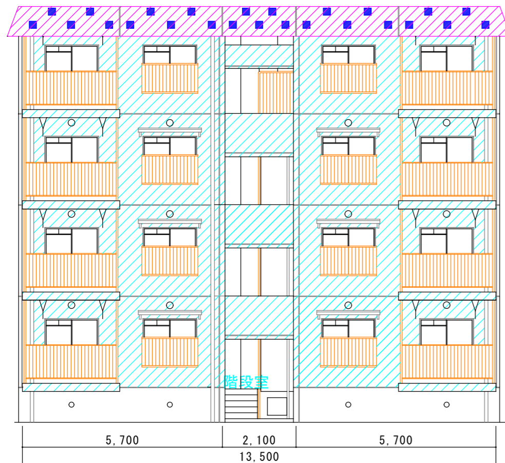
B棟 正面図
