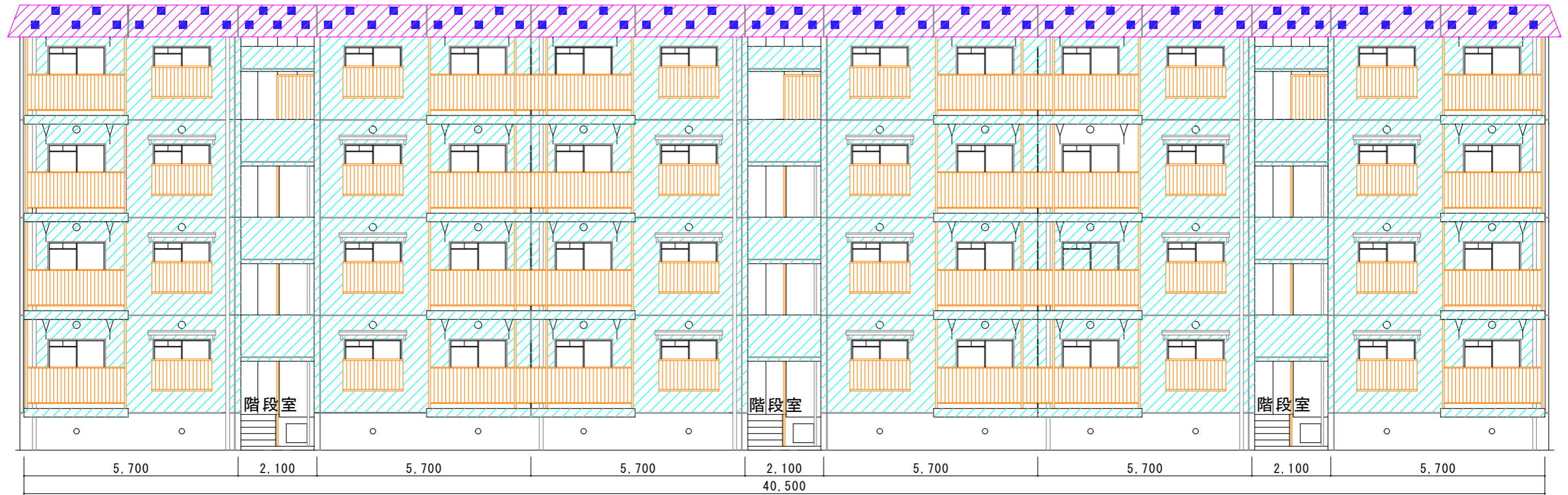
A棟 正面図
