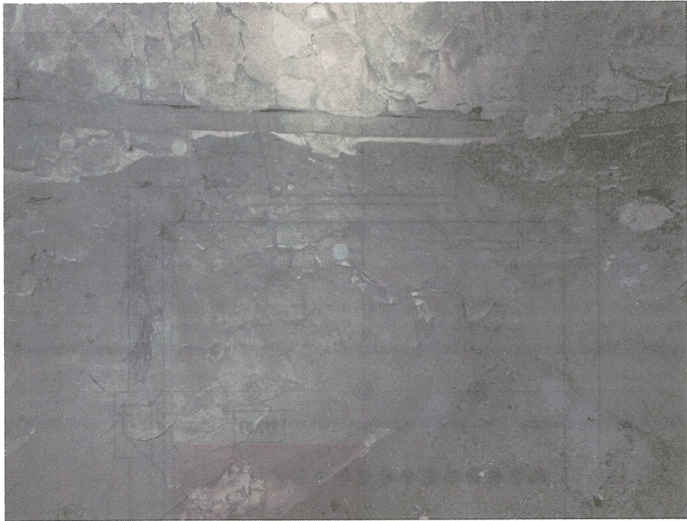
反助燃バーナ側耐火物 損傷状況
