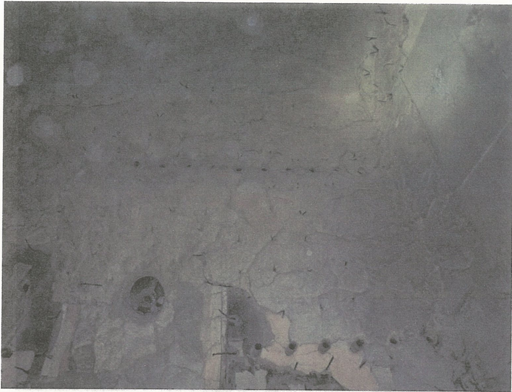
助燃バーナ側耐火物 損傷状況
